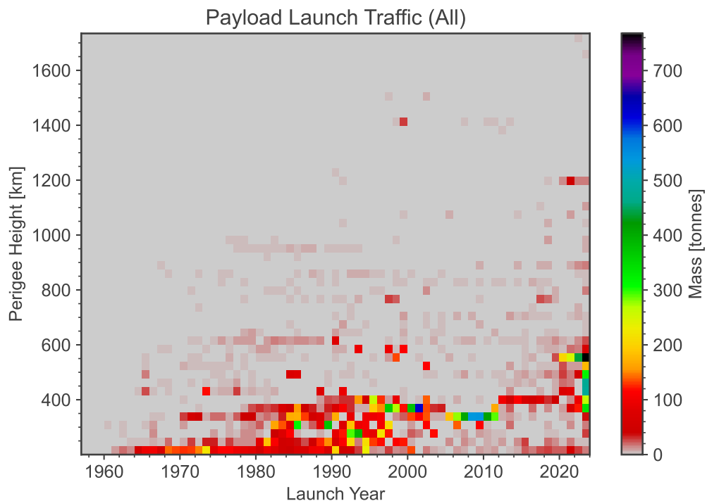
(a) LEO IADC
